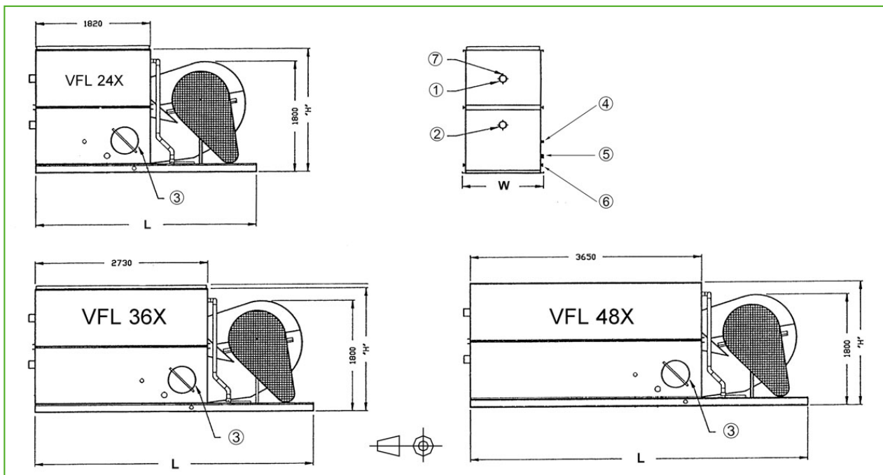
1. Впуск воды НД 100; 2. Выпуск воды НД 100; 3. Дверца люка; 4. Подпитка НД 25; 5. Перелив НД 50 для VFL 24x - VFL 36x и НД 80 для VFL 48X; 6. Слив НД 50; 7. Вентиляционный канал НД 15.
